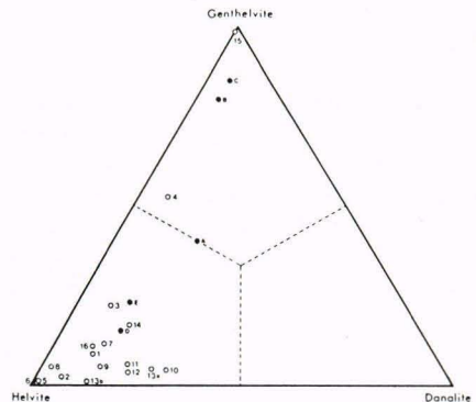
Fig. 1 Helvin-danalitt-genthelvin diagram.
