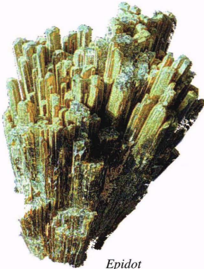
Epidot
