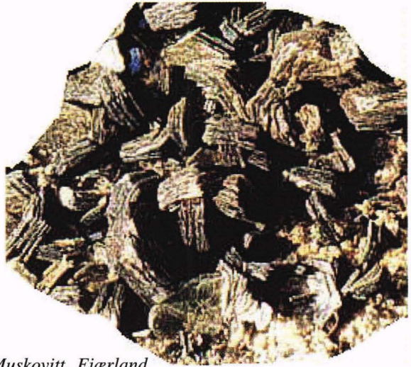
Muskovitt, Fjærland
